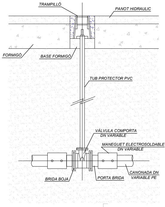
VÀLVULA DE COMPORTA AMB EIX DE COMANDAMENT
