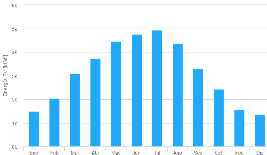
Figura 6. Producció anual d'energia sistema fotovoltaic (Camp 1).
