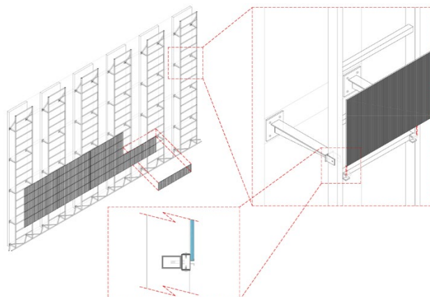
Figura 3. Sistema de fixació captadors al perfil.
