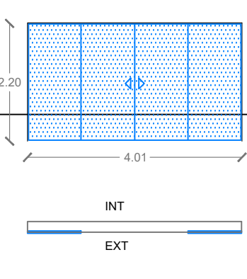
P1 PORTA D'ACCÉS UNITATS:1
