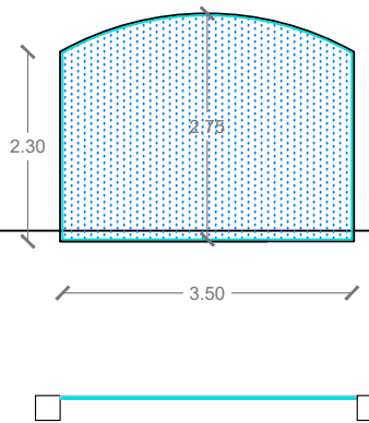
F2 FINESTRAL UNITATS:2
