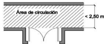
Figura 1.1 Disposición de puertas laterales a vías de circulación
