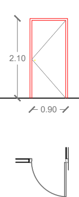
P4 PORTA BATENT UNITATS:1
