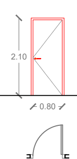
P6 PORTA BATENT UNITATS:2
