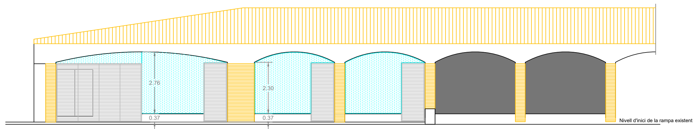
ALÇAT PROPOSTA. C-C'
