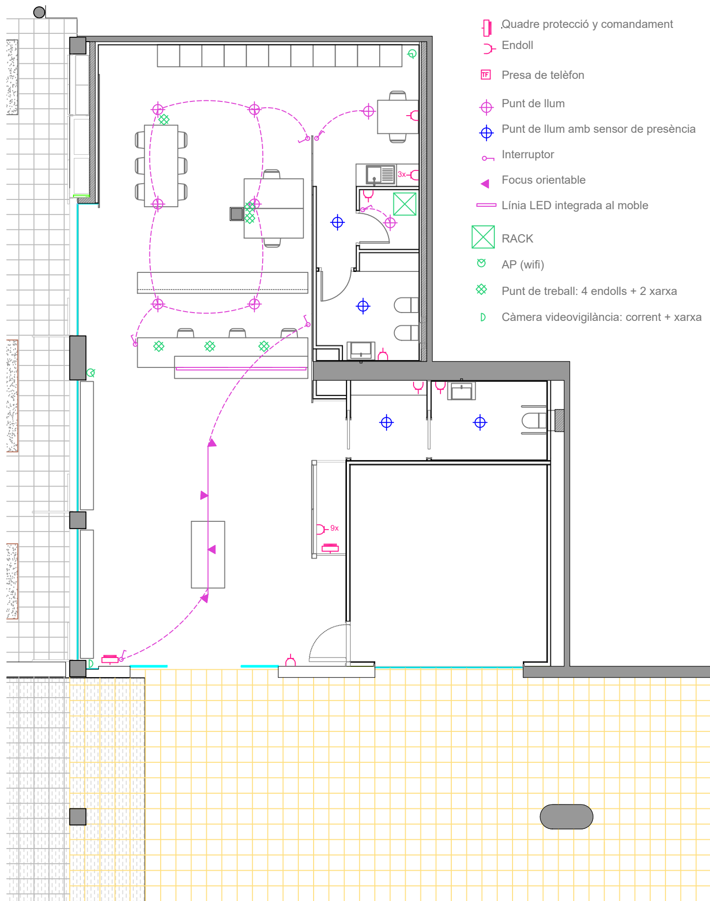
INSTAL·LACIONS D'ELECTRICITAT, ENLLUMENAT I TELEFONIA
