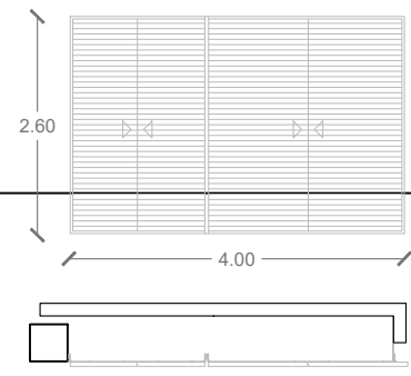
P3 PORTA DE SERVEIS UNITATS:1
