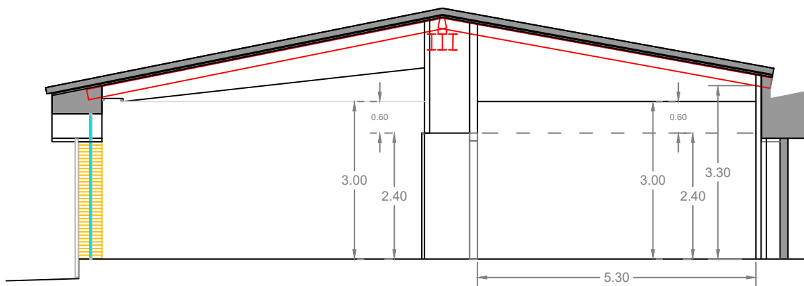
SECCIÓ PER LA SALA IMMERSIVA. B-B'
