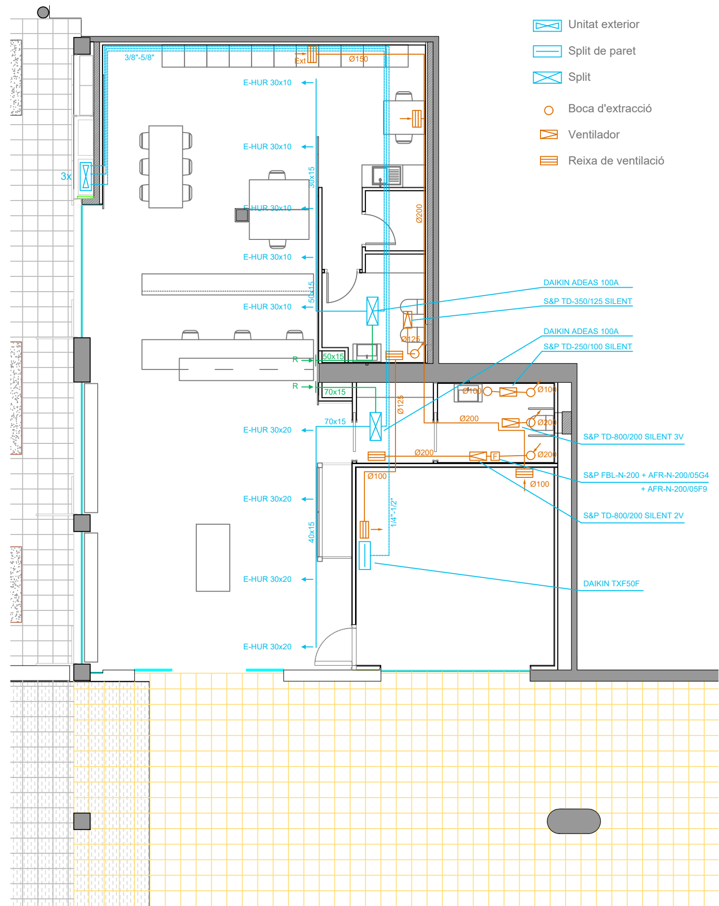
INSTAL·LACIONS DE CLIMATITZACIÓ
