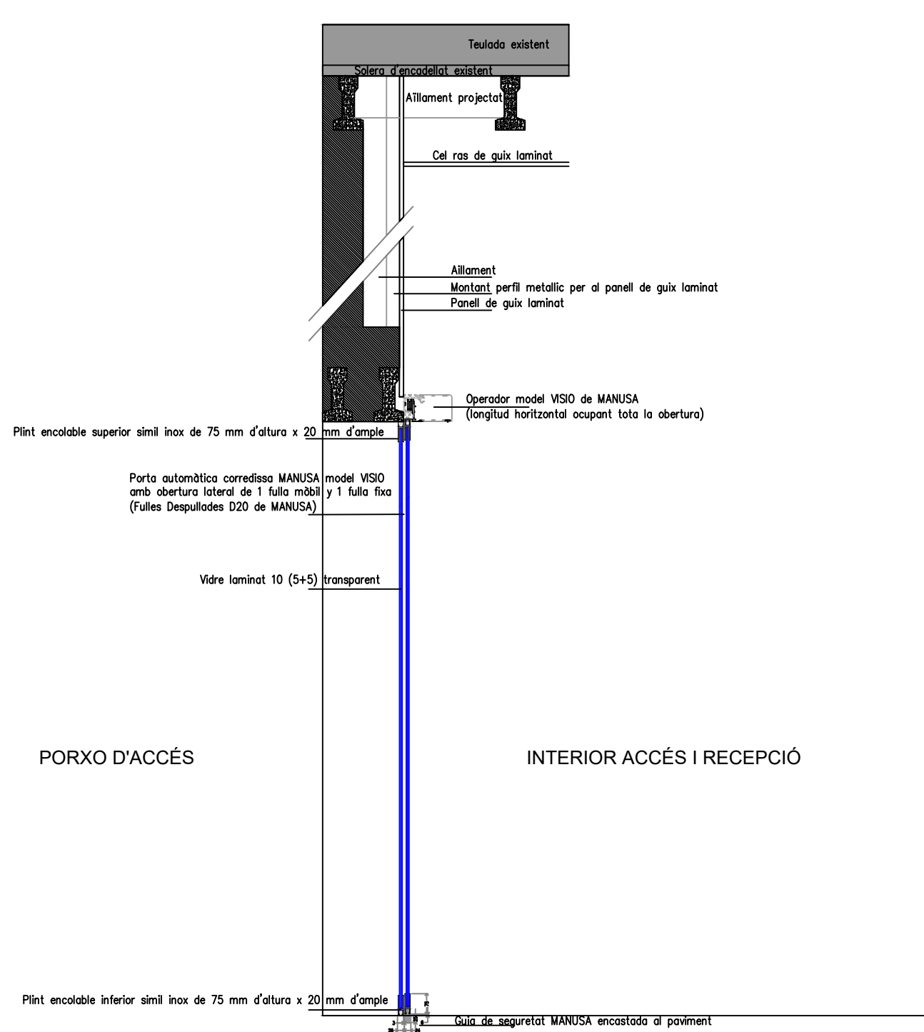
DETALL CONSTRUCTIU DE LA PORTA D'ACCÉS
